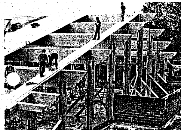
Toiture porteuse
