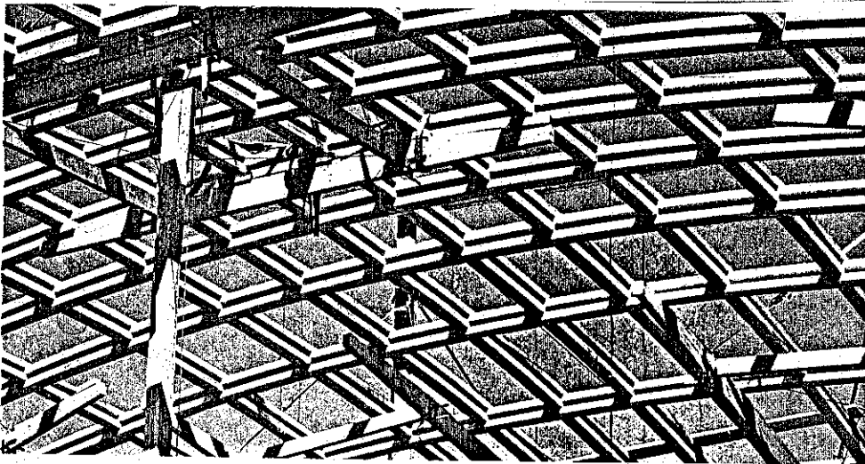
Halle de tennis. Structure en bois lamellé-collé industriel monté au sol. Courbure obtenue par fléchissement naturel de la charpente lors de son élévation par le centre.
